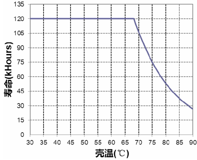
寿命 vs. 壳温
