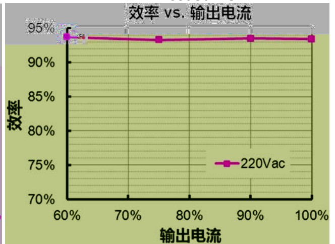
EBV-350S048SV 效率 vs. 输出电流
