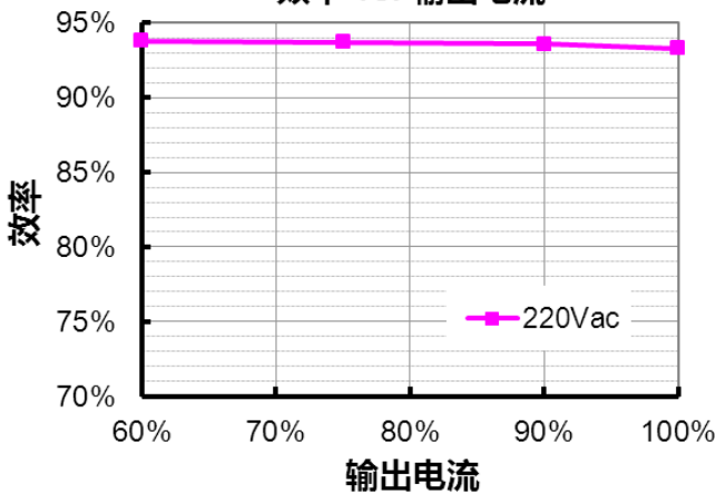
EBV-400S036SV 效率 vs. 输出电流
