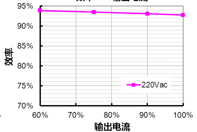
EBV-400S048SV 效率 vs. 输出电流
