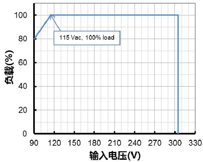
降额曲线
