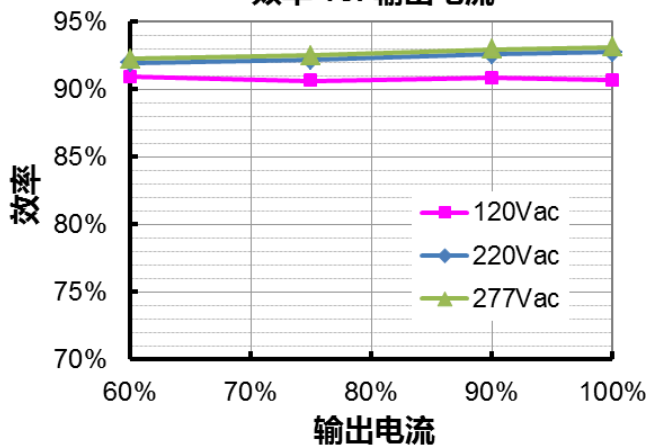
EUV-600S048SV 效率 vs. 输出电流
